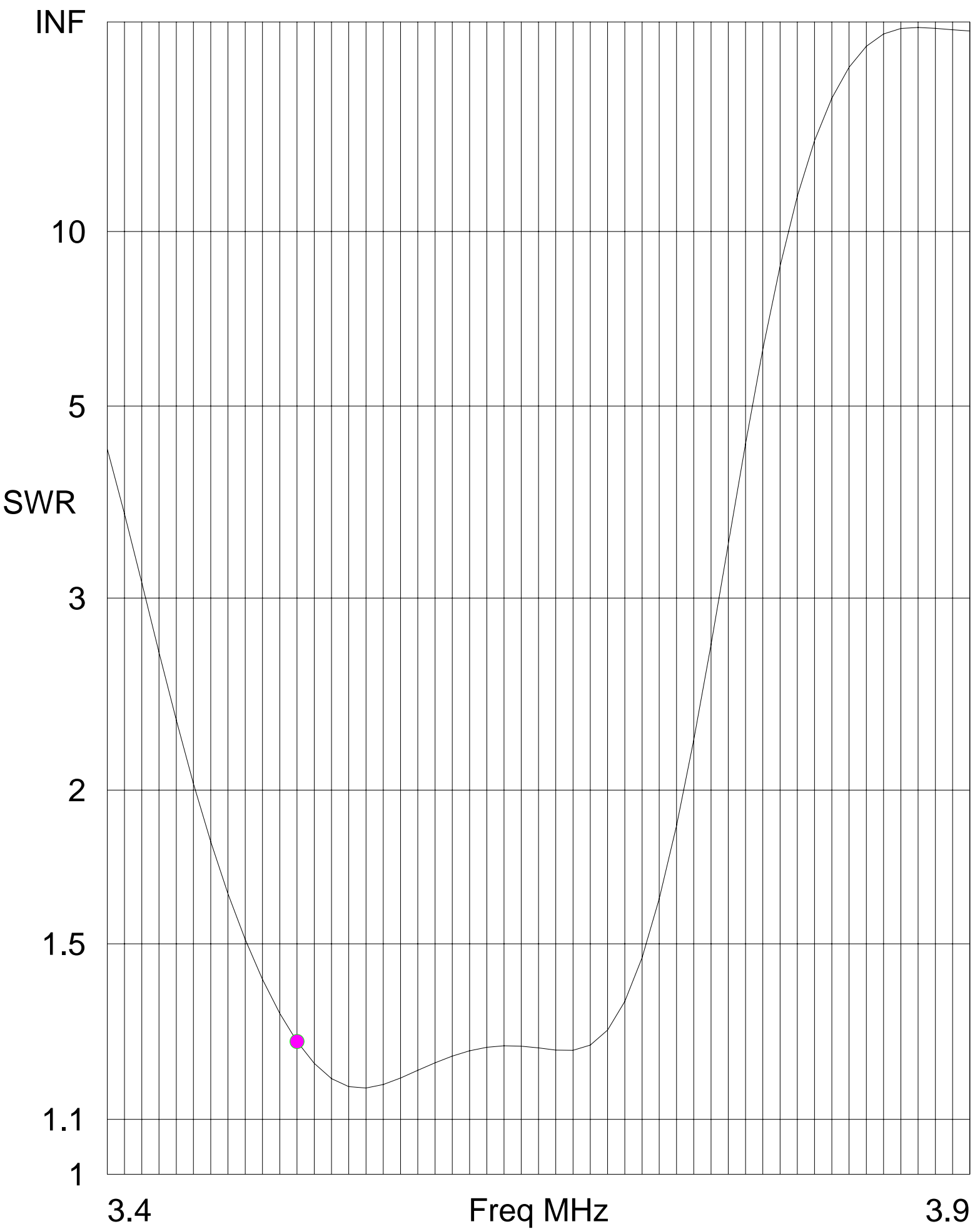
80m owa80jy5 EZnec
